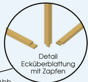
Abb. Konstruktion mit Fundamentrahmen
