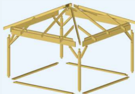
image Assemblage tenon et mortaise image construction avec châssis de fondation
